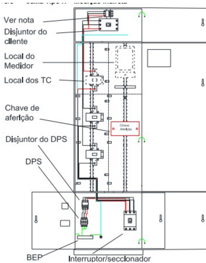
Figura 2 - Caixa H - Medição Indireta (página 75 da GED 13)
