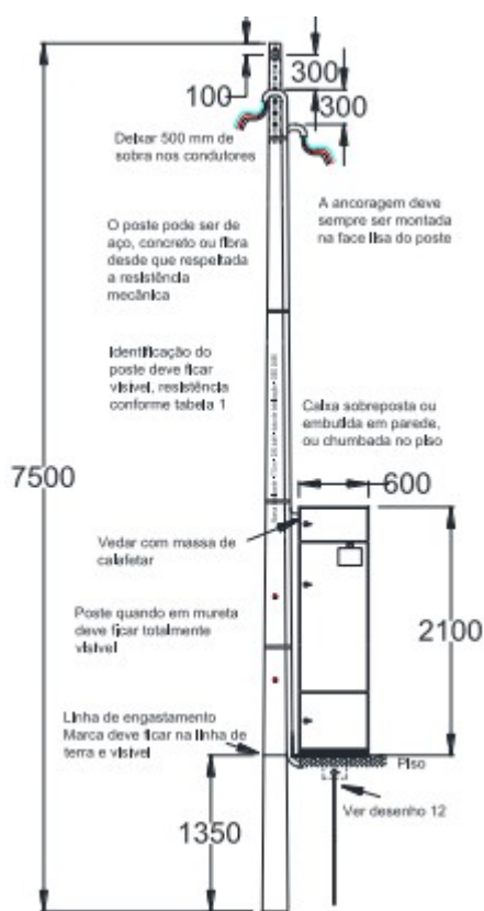
Figura 1- Caixa H - Forma de Instalação (página 73 da GED13 CPFL)
