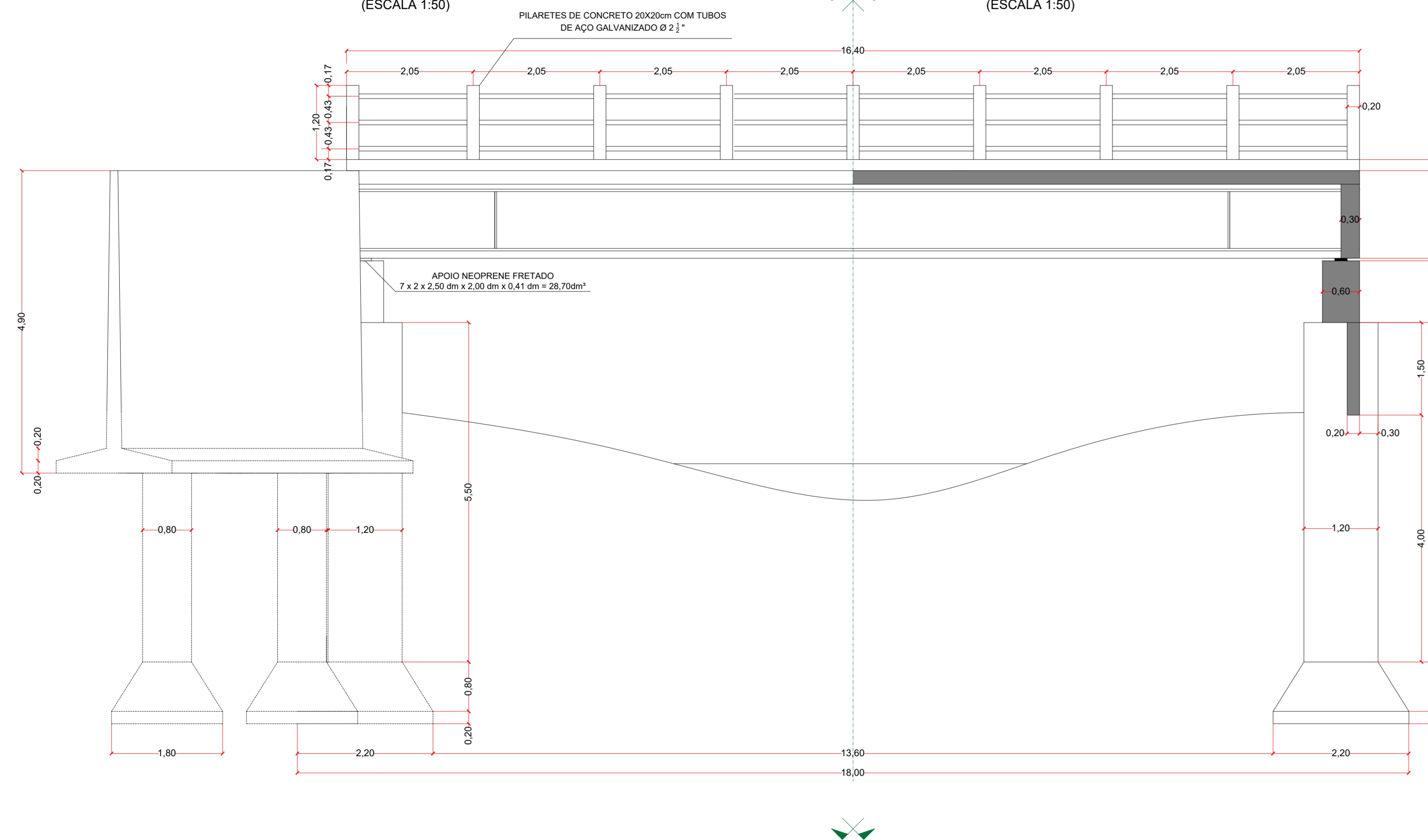
1/2 VISTA LONGITUDINAL (ESCALA 1:50)
