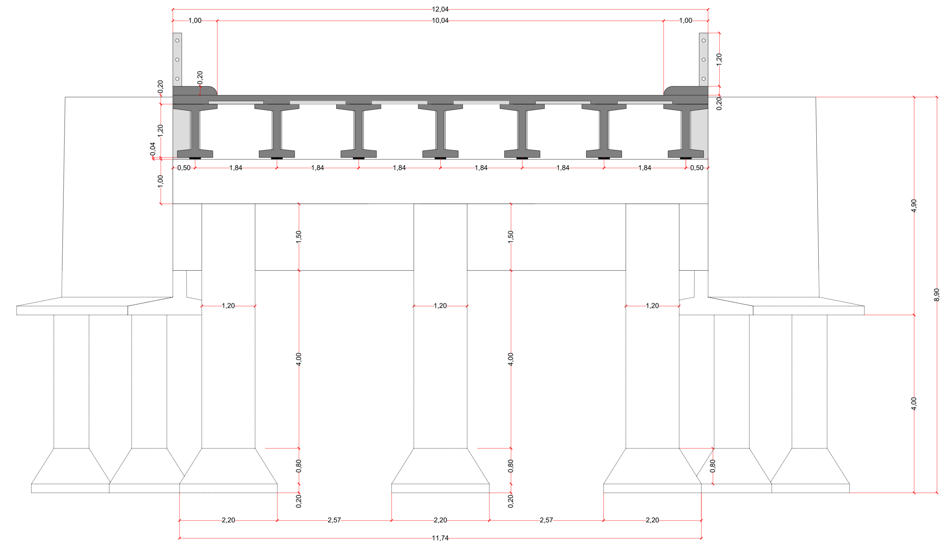
CORTE TRANSVERSAL (ESCALA 1:50)
