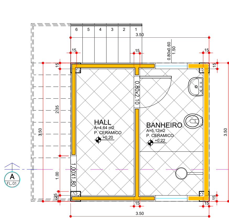
PLANTA - PAV. INFERIOR ESCALA 1:50
