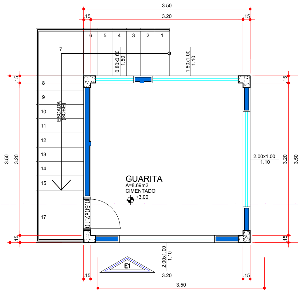
PLANTA - PAV. SUPERIOR ESCALA 1:50
