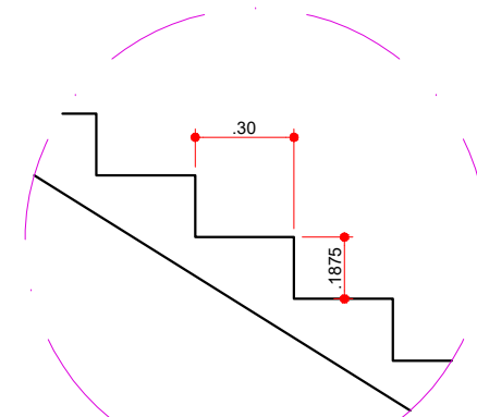
DETALHE DA ESCADA ESCALA 1:25
