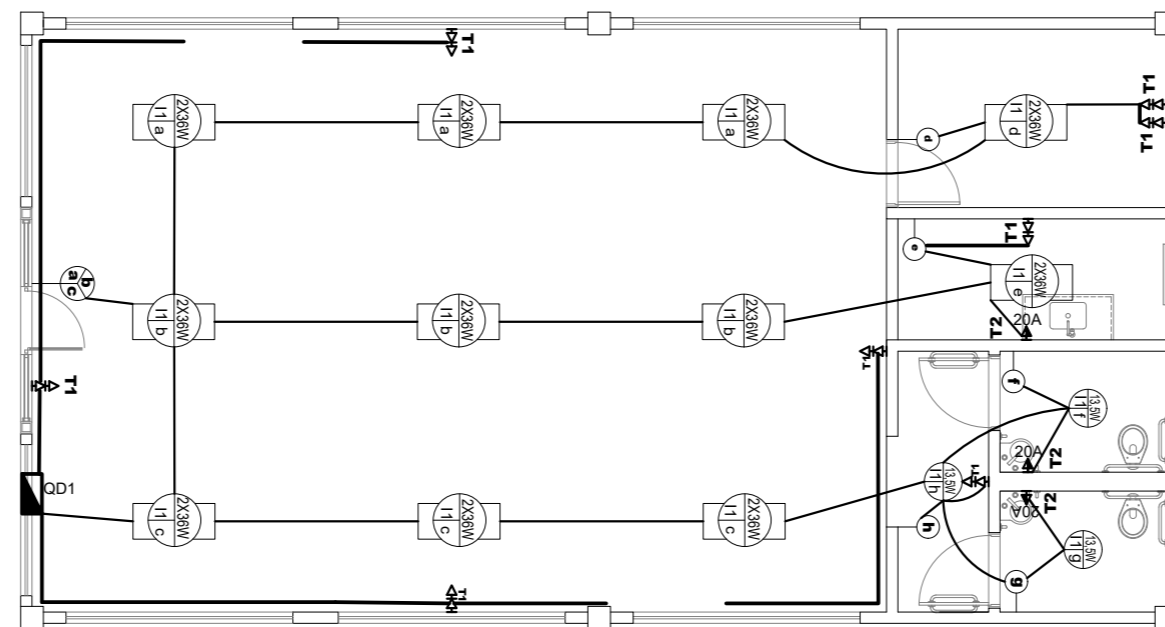
PLANTA ESC. 1:100
