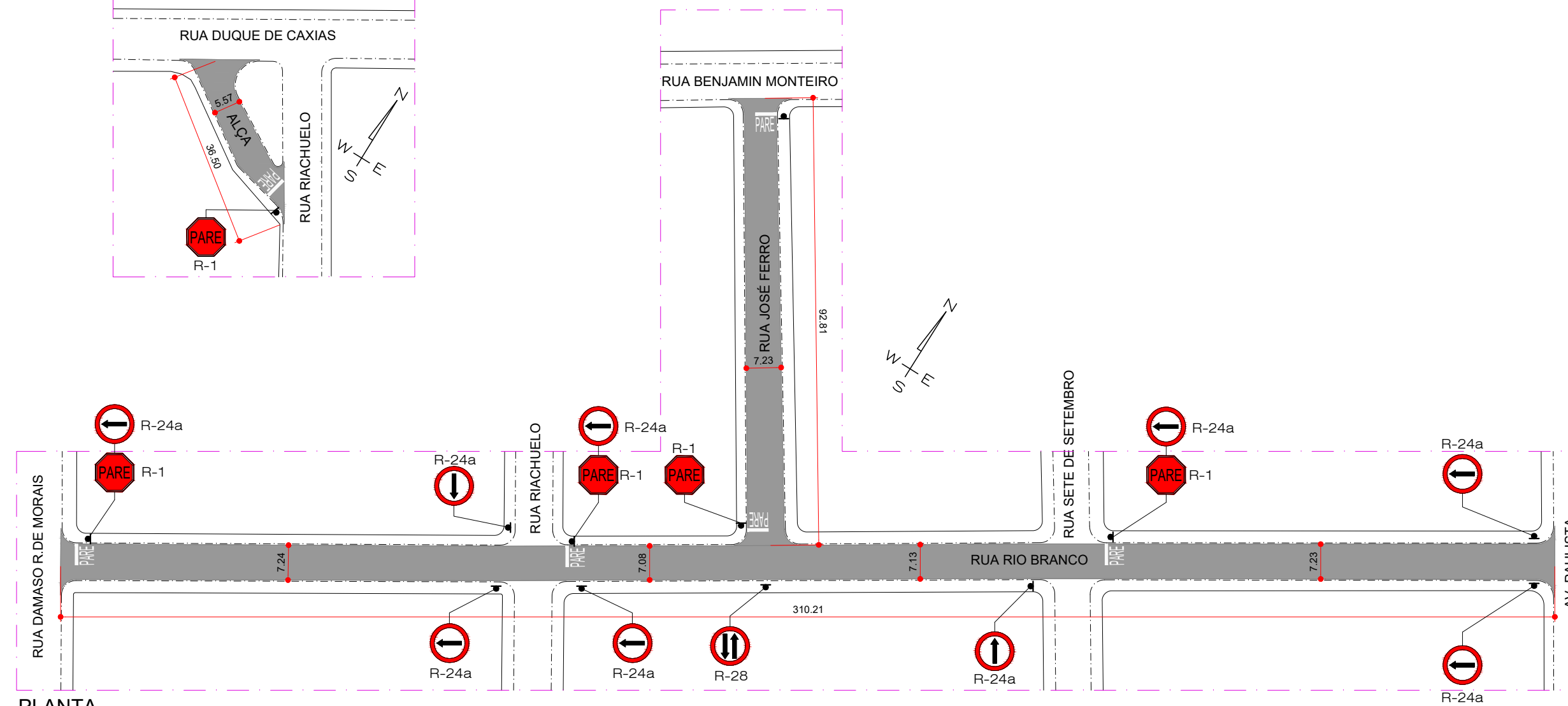
PLANTA ESC. 1:1.000
