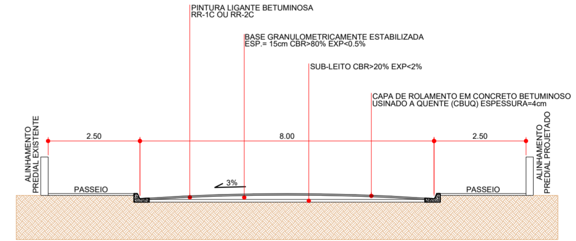
VIA A PAVIMENTAR - PERFIL TRANSVERSAL S/ ESCALA
