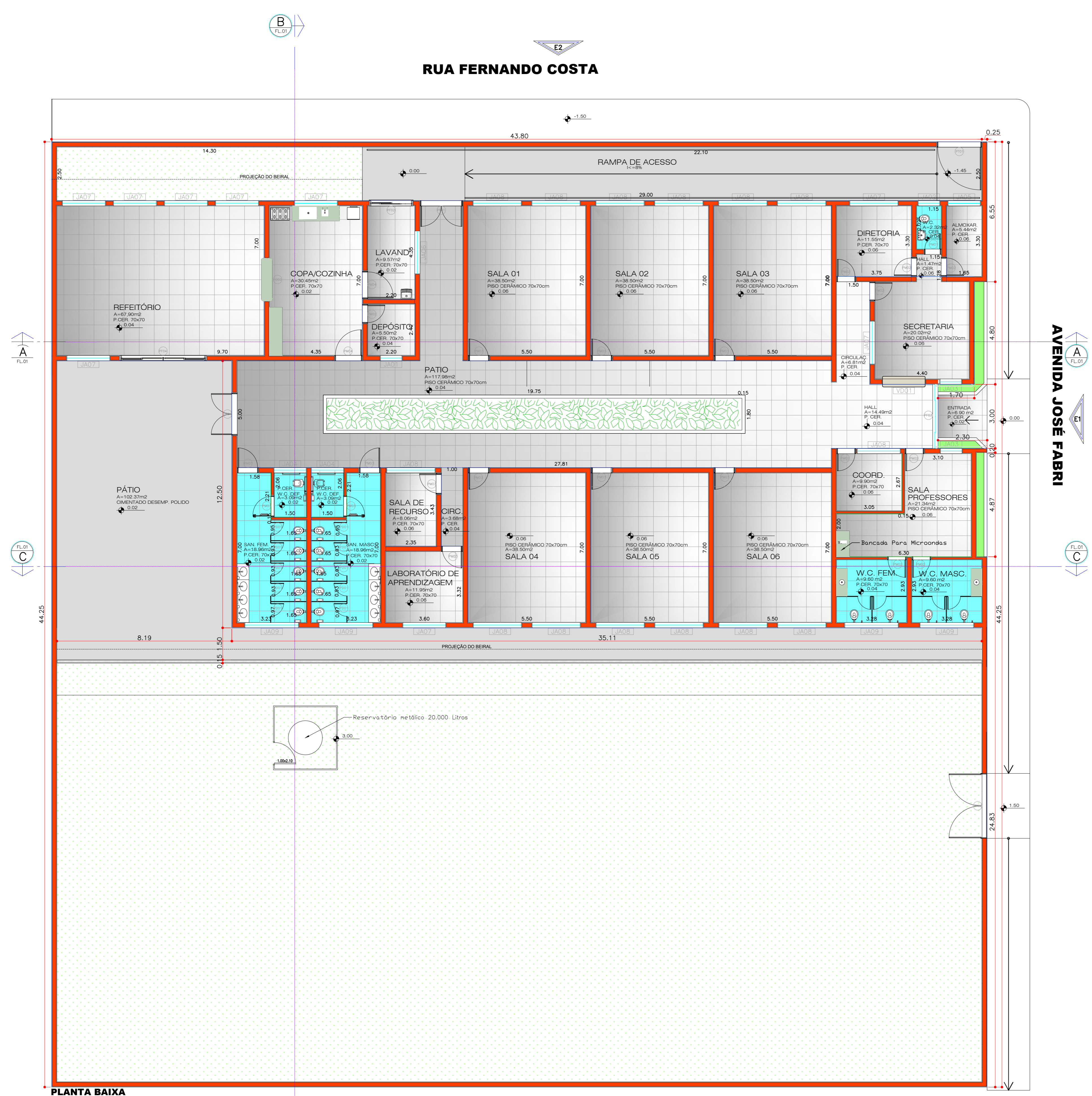
PLANTA BAIXA ESC 1:100
