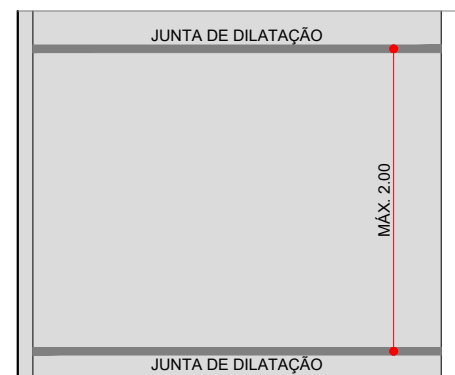
DETALHE DA JUNTA DE DILATAÇÃO ESC. 1:50 QUANTIDADE: 820.00m
