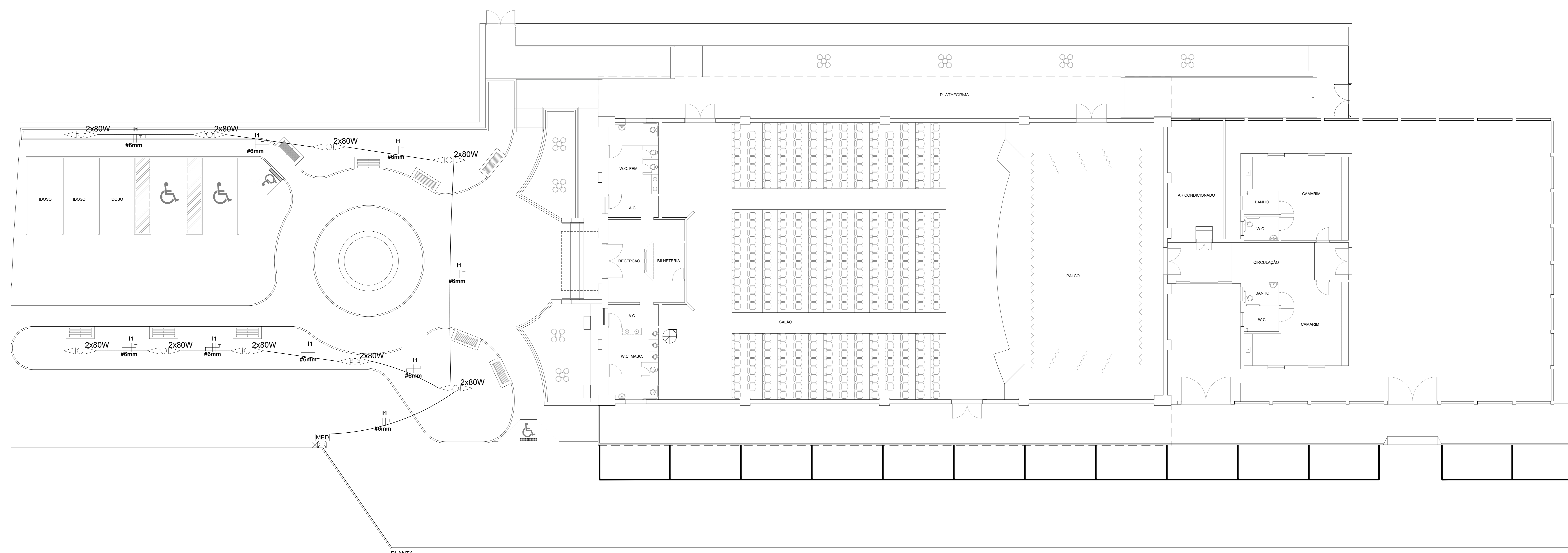
PLANTA ESC 1:100
