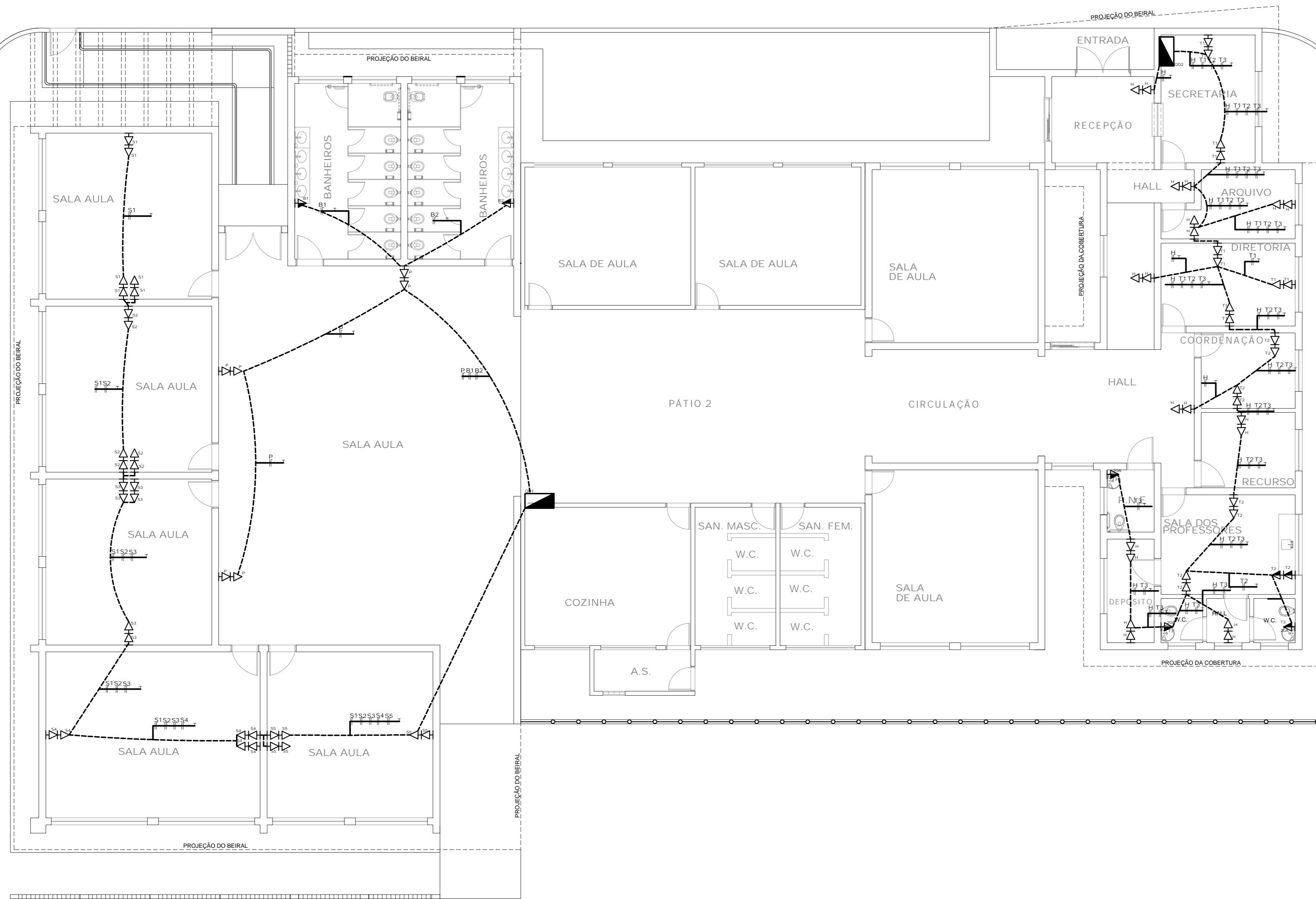
PLANTA - ILUMINAÇÃO ESC 1:100
