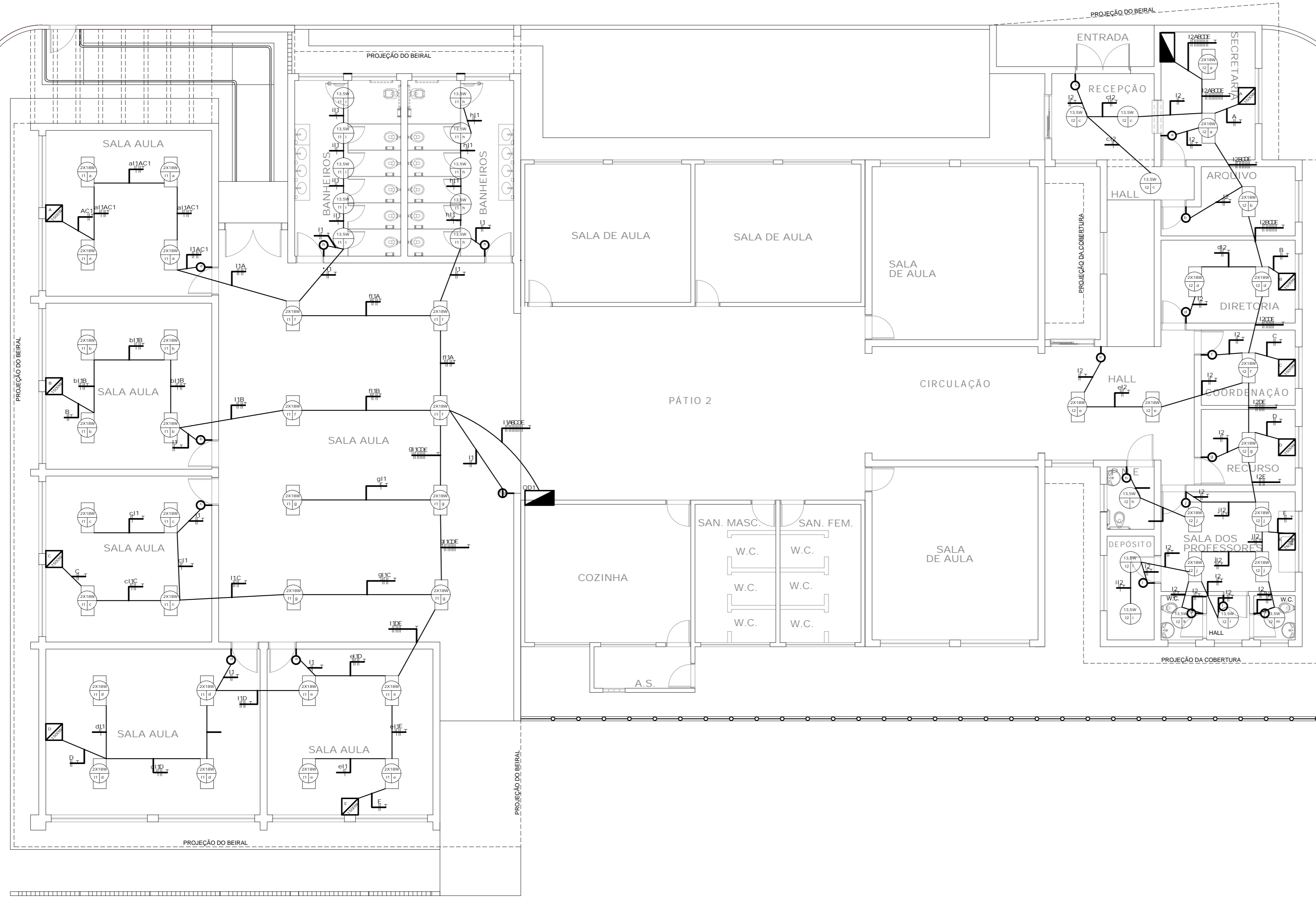
PLANTA - ILUMINAÇÃO, AR CONDICIONADO ESC 1:100
