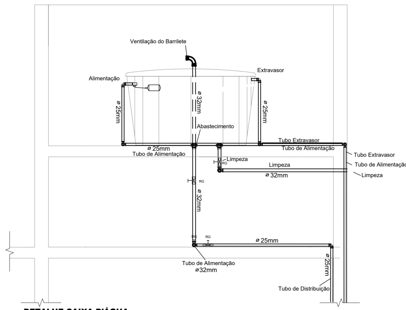
DETALHE CAIXA D'ÁGUA ESC. 1:25
