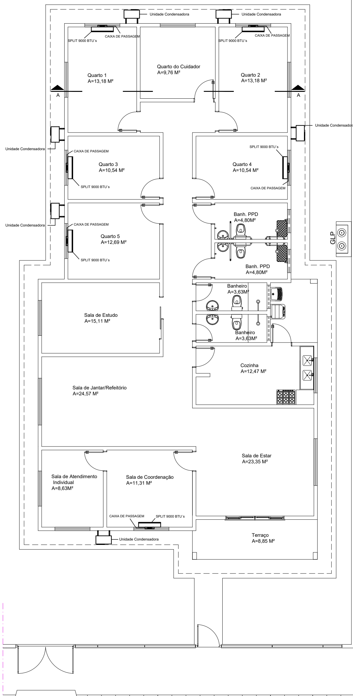
PLANTA ESC 1:100
