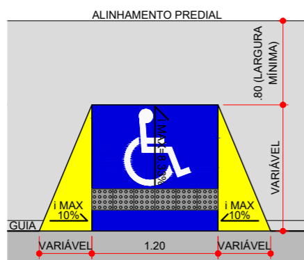
RAMPA DE ACESSO P/ P.N.E. ESC. 1:50
