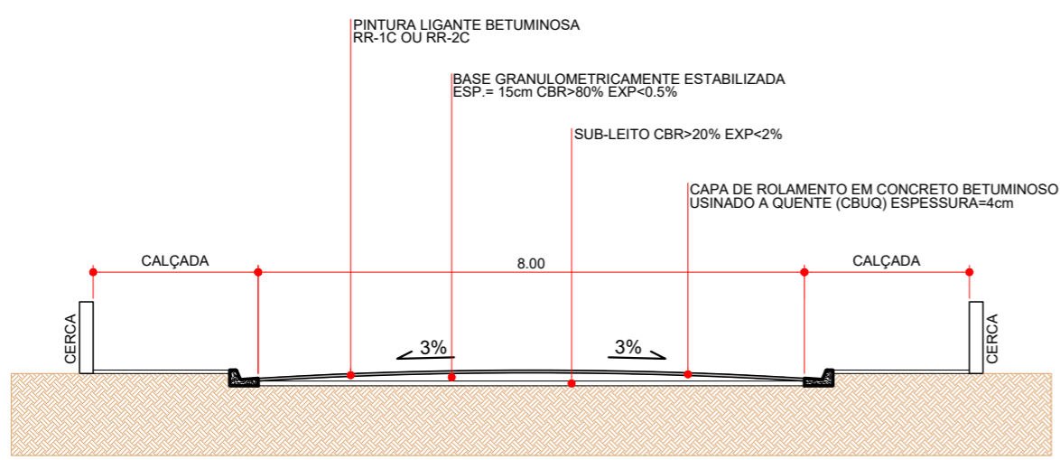
PERFIL TRANSVERSAL ESC. 1:100
