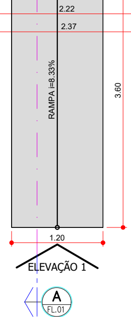
PLANTA ESCALA 1:50
