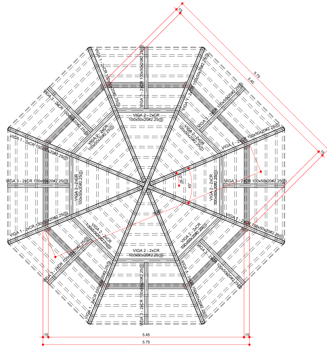
PLANTA VISTA SUPERIOR ESCALA 1:25
