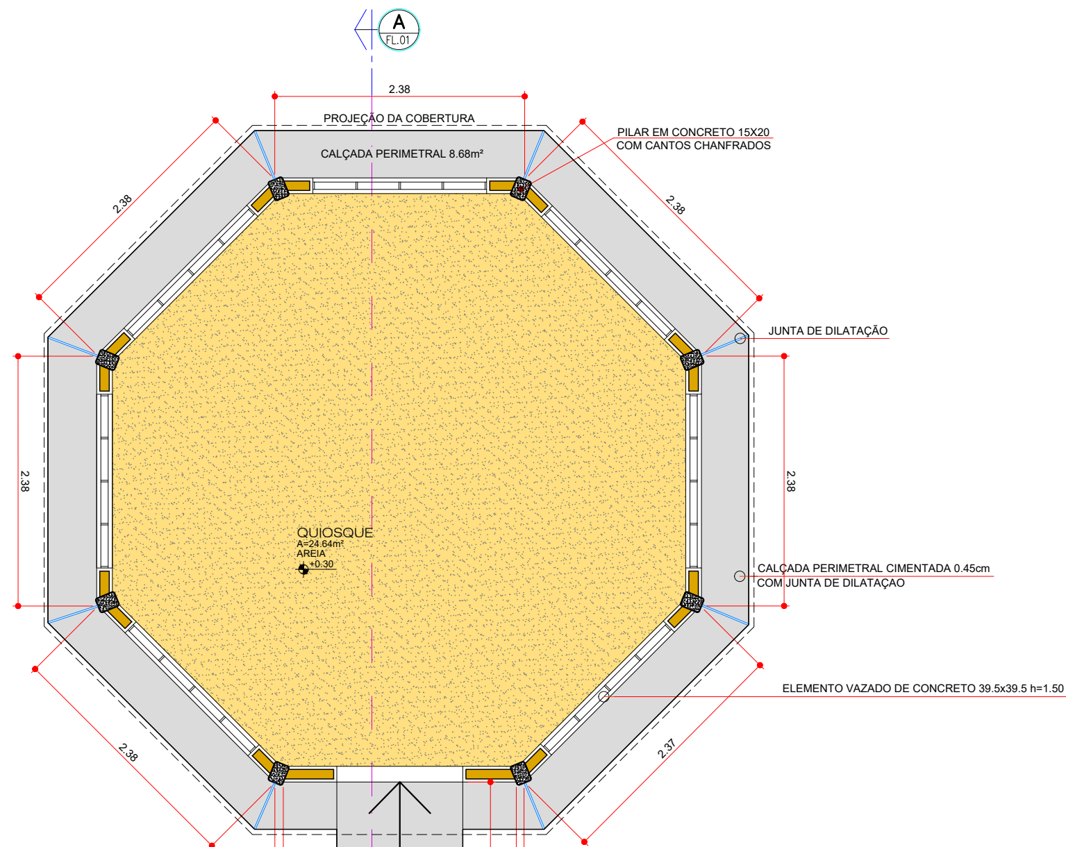
PLANTA ESCALA 1:50
