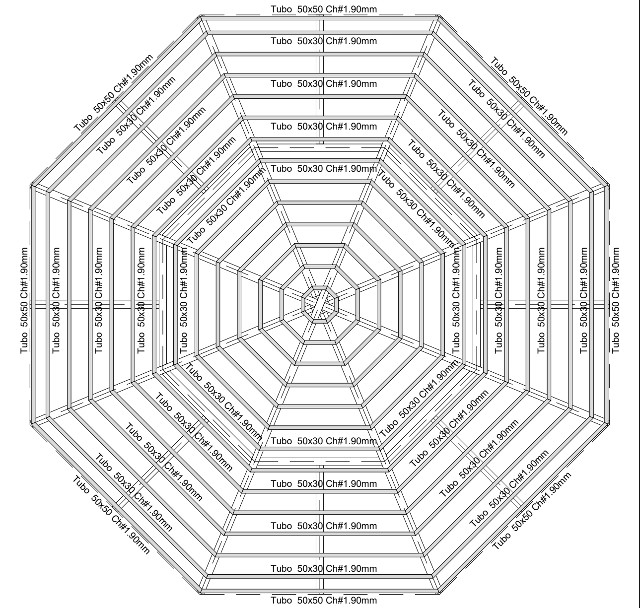
PLANTA VISTA SUPERIOR RIPAS ESCALA 1:25
