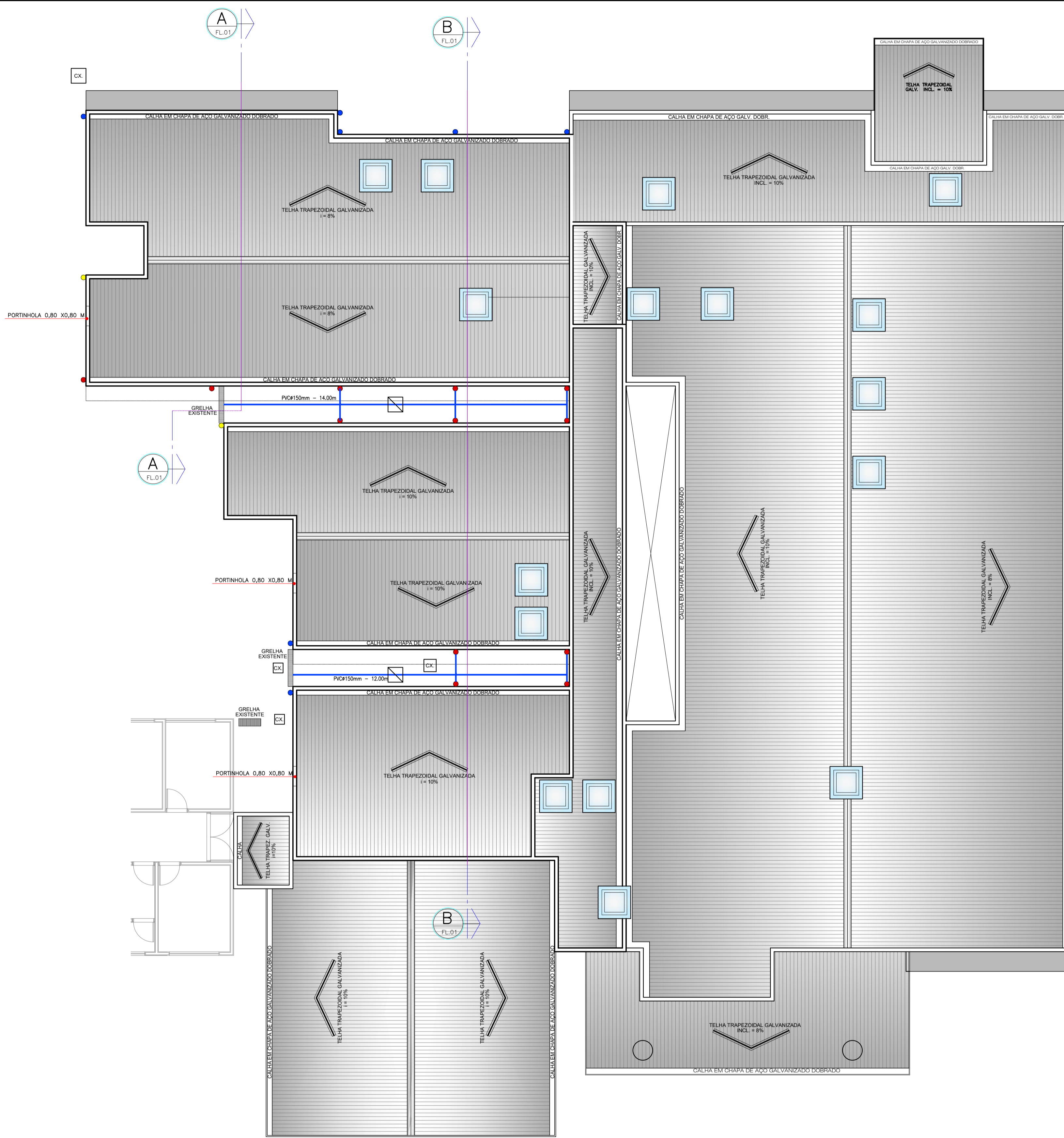
PLANTA DE COBERTURA - IMPLANTAÇÃO ESC 1:100
