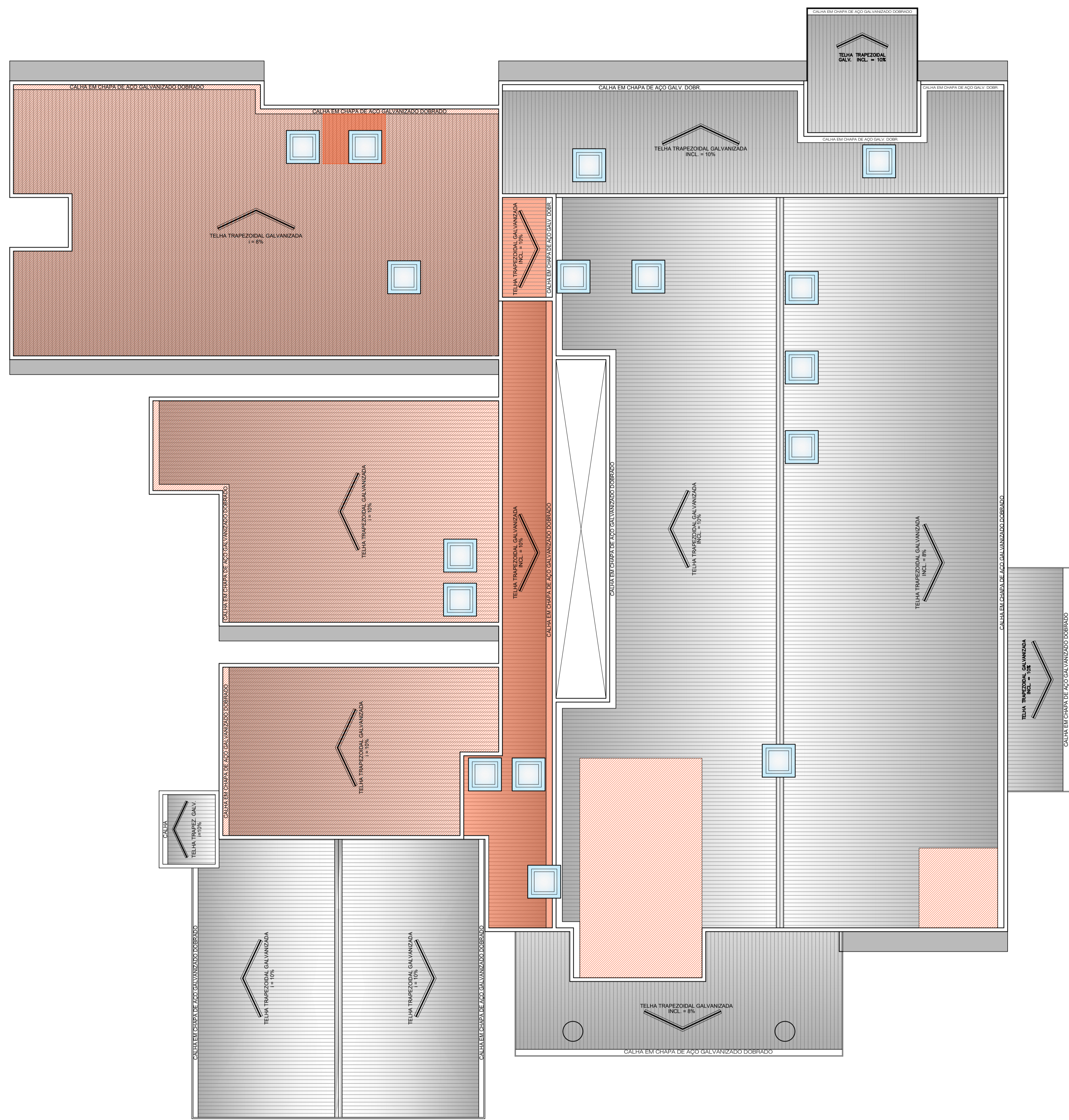
PLANTA DE COBERTURA - SITUAÇÃO ESC 1:100
