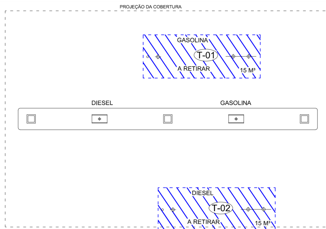
PLANTA BAIXA - ATUAL ESCALA 1:100
