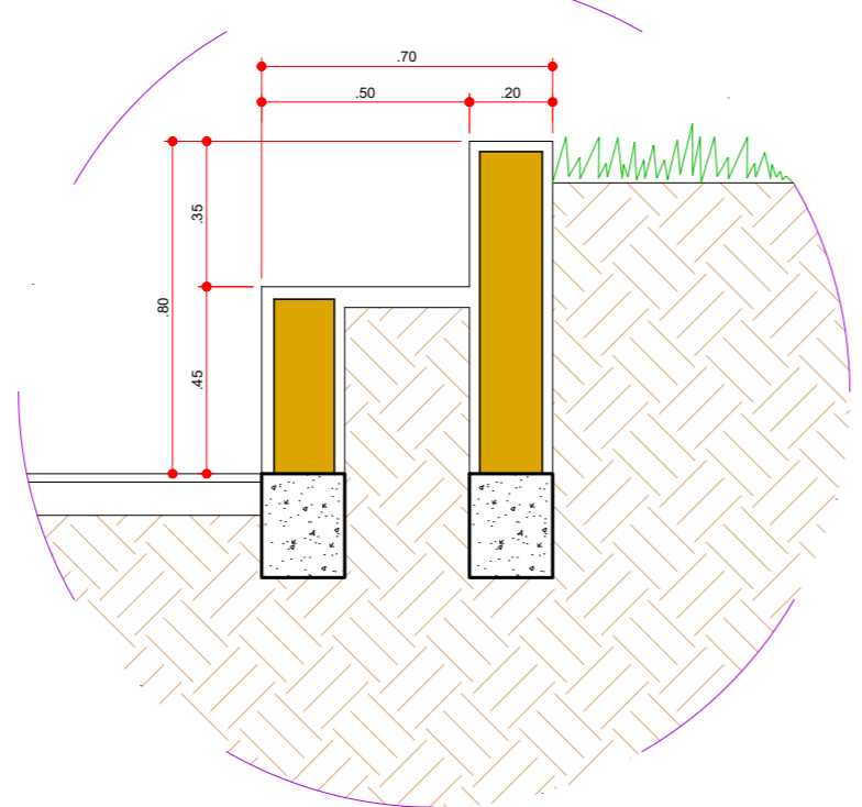
CORTE DA ARQUIBANCADA ESC. 1:20
