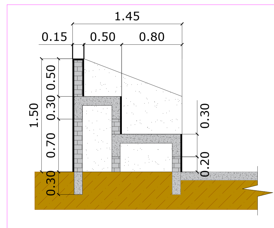
CORTE DA ESCADA S/E
